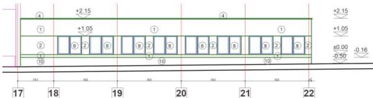
Fasadă principală - releveu:
